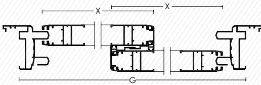
A-A KESİTİ / SECTION
