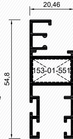
Sineklik Çıta Profili - Fly Screen Beat Profile
