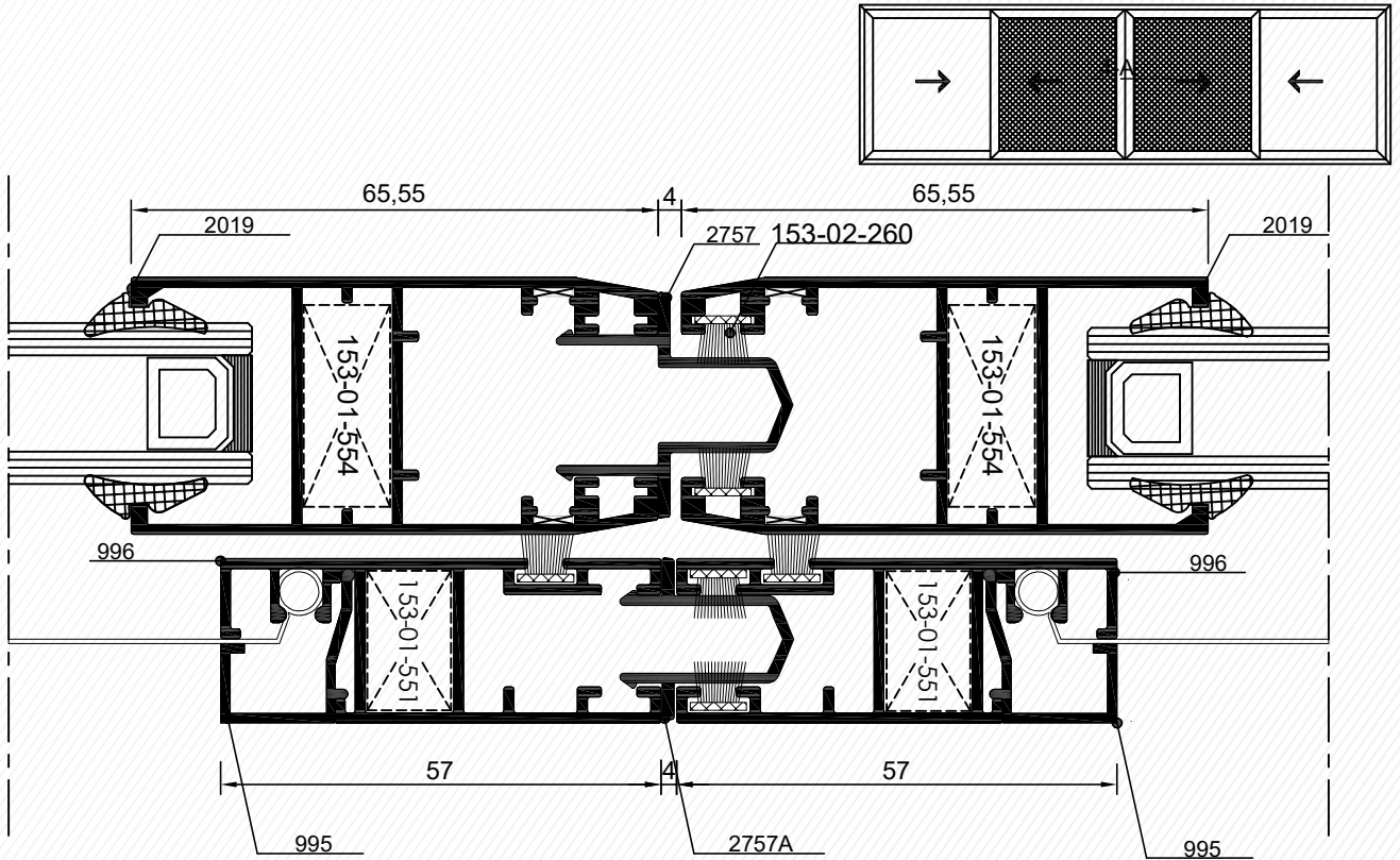
4-A DETAYI DETAIL
