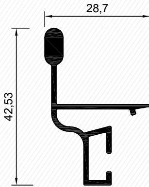
Sineklik Çıta Profili - Fly Screen Beat Profile
