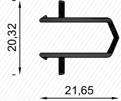
Sineklik Adaptör Profili Fly Screen Adapter Profile
