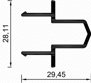
Adaptör Profili - Adapter Profile
