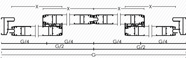
A-A KESİTİ / SECTION
